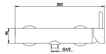
Cod. 32552CR0EPR Miscelatore doccia esterno External shower mixer
