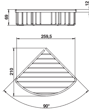
Cod. 30011CRPR Cestello singolo ad angolo Corner basket soap holder
