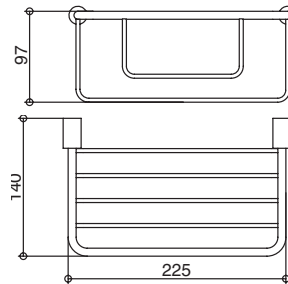
Cod. 30017CRPR Cestello rettangolare Rectangular basket
