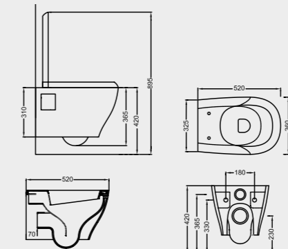
MW10 WC SOSPESO FUNZIONA CON 4,5 LITRI WALL-HUNG WC NOMINAL FLUSH 4,5 LITERS
