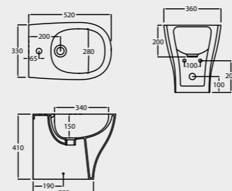
M24 BIDET A TERRA - INSTALLAZIONE FILO PARETE FLOOR MOUNTED BIDET - BACK TO WALL INSTALLATION
