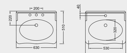
D19 LAVABO 63 + D16 COLONNA WASHBASIN 63 + PEDESTAL
