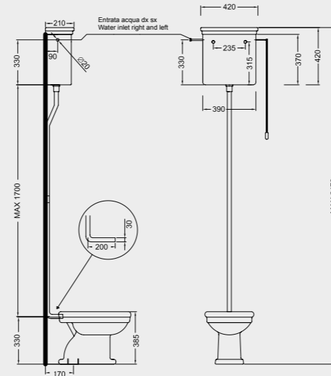
D50 CASSETTA ALTA + D59 CASSETTA ALTA CON COPERCHIO HIGH CISTERN + HIGH CISTERN WITH LID
