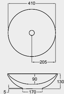
A42 LAVABO D'APPOGGIO POLIS 41x41x13 POLIS COUNTERTOP WASHBASIN 41x41x13
