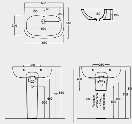
M15 LAVABO 65 APOGGIO / DA COLONNA + M16 COLONNA PER LAVABI + M22 SEMICOLONNA COUNTER TOP / WASHBASIN FOR PEDESTAL 65 + PEDESTAL FOR WASHBASIN + SEMIPEDESTAL
