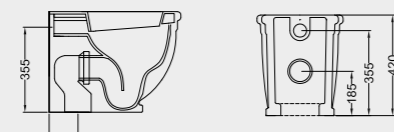
QUOTE PER IMPIANTI ESISTENTI INSTALLATION ON EXISTING IMPLANTS
