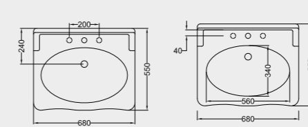
D15 LAVABO 68 + D16 COLONNA WASHBASIN 68 + PEDESTAL
