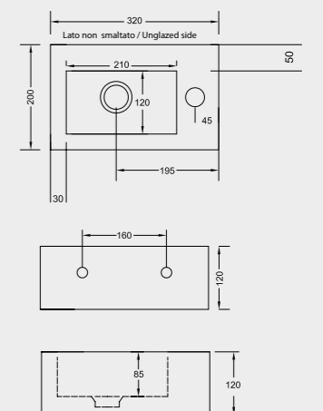
LO20 LAVABO DA APPOGGIO / SOSPESO WALL HUNG / COUNTERTOP WASHBASIN
