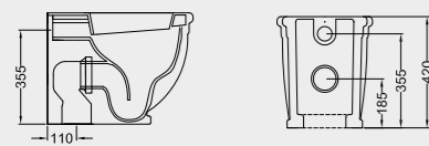
QUOTE NUOVI IMPIANTI INSTALLATION ON NEW IMPLANTS
