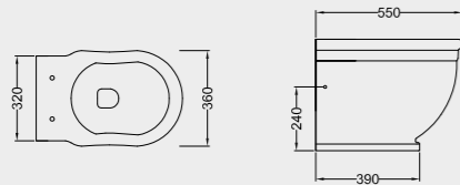
QUOTE NUOVI IMPIANTI INSTALLATION ON NEW IMPLANTS
