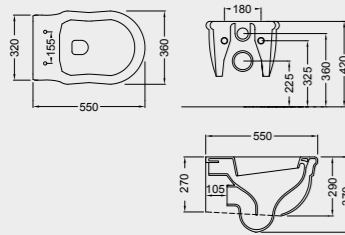
DW10 VASO SOSPESO WALL-HUNG WC
