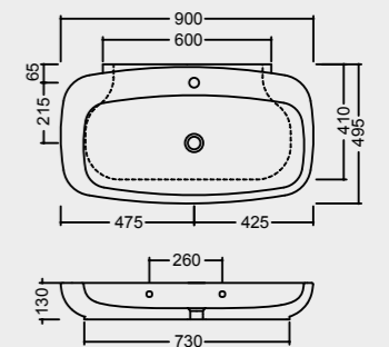
DL52 LAVABO 90 APPOGGIO / SOSPESO COUNTERTOP / WALL-HUNG WASHBASIN 90
