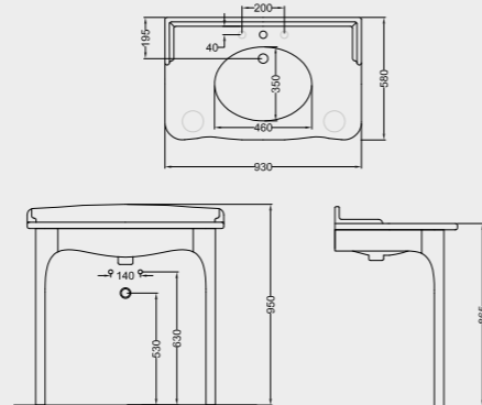
D99 STRUTTURA LEGNO NERA + CONSOLLE 93 BLACK WOOD FURNITURE + CONSOLLE 93
