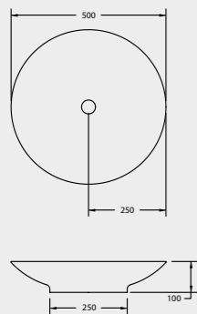
A24 SOUL 500 REI LAVABO TONDO D'APPOGGIO 50x50x10 SOUL 500 REI COUNTERTOP ROUND WASHBASIN 50x50x10
