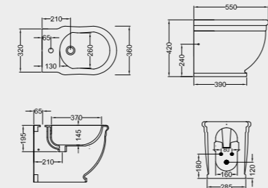
D24 BIDET FILO MURO BIDET BACK TO WALL
