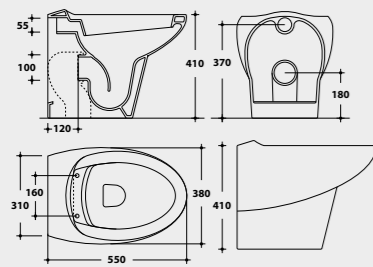
TAW14 BIDET SOSPESO WALL HUNG BIDET
