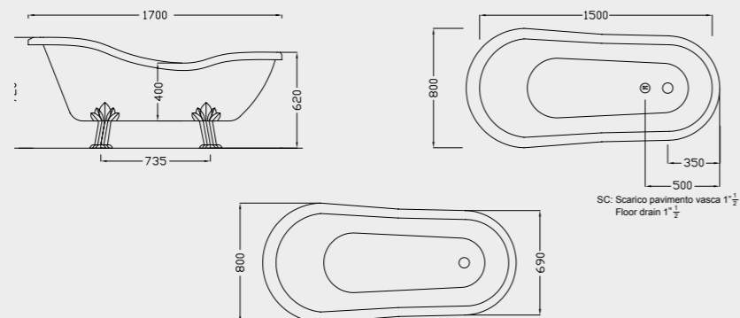
D60 - D61 - D62 - D63 VASCA BATHTUB
